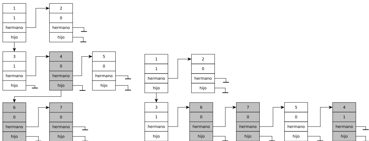
(a) Arbol previo a arbolizar el nodo de color con valor 4.
